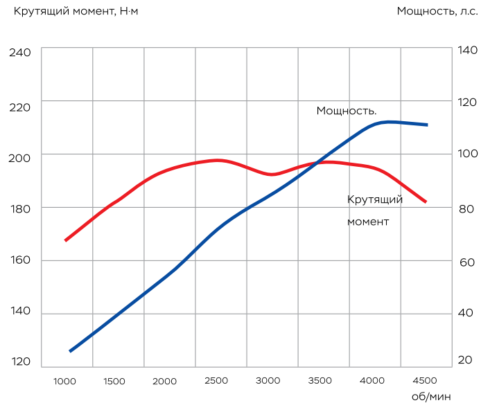
График для двигателя ЗМЗ-40911
